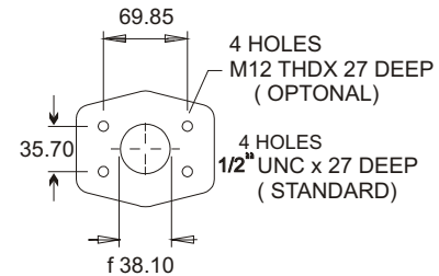
1-1/2" SAE FLANGE
